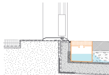
Seuil de porte perméable
