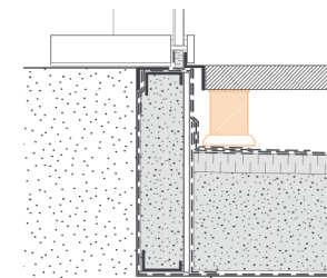
Dallage sur plots
